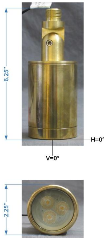
FIG. 1 LUMINAIRE
