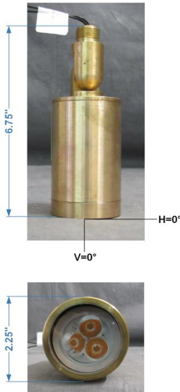
FIG. 1 LUMINAIRE
