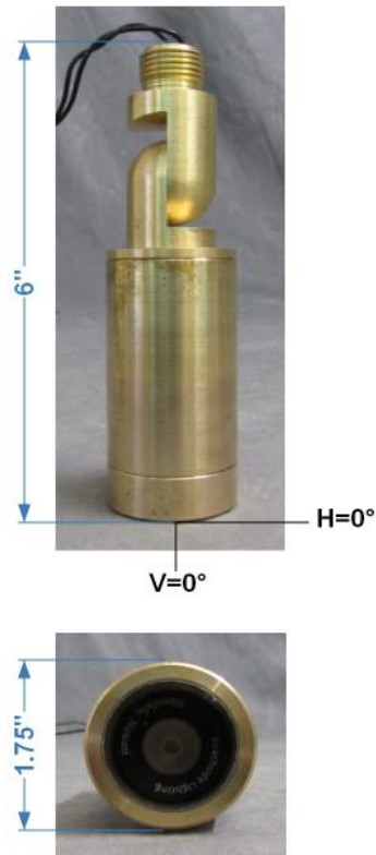
FIG. 1 LUMINAIRE
